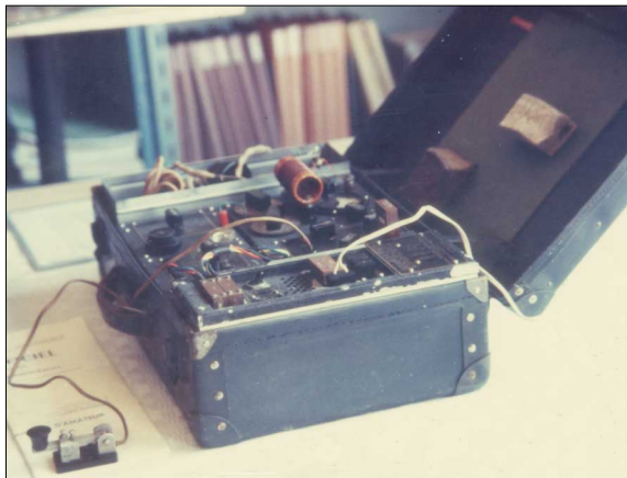
Valise utilisée, pendant la dernière guerre, par les opérateurs de la Résistance
