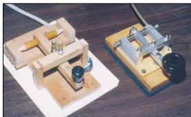
Manipulateurs de télégraphie (morse)
